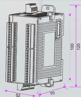
Fig. A FlexiLogics® controller module
